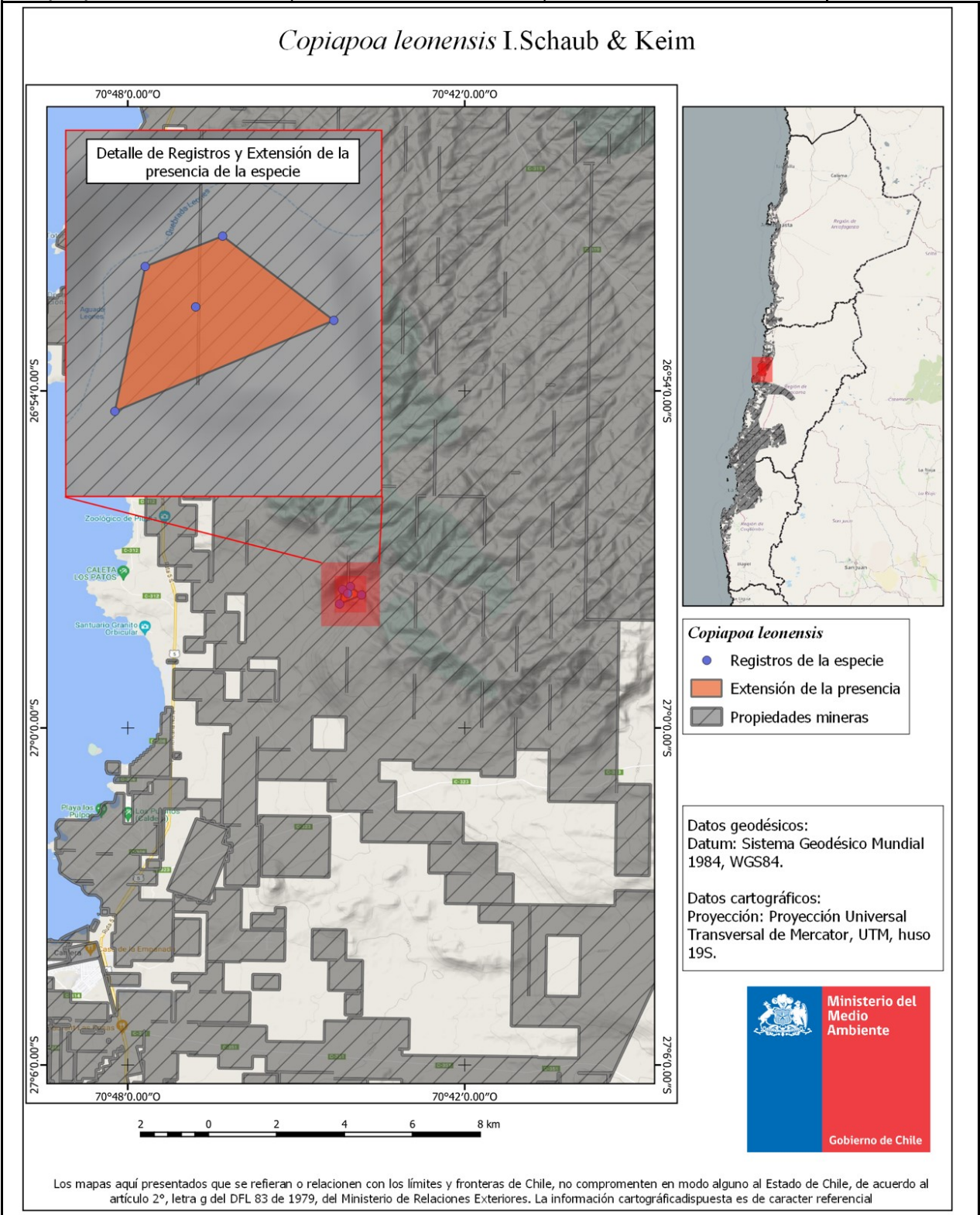
Figura 4. Mapa de registros (ocurrencias) y extensión de presencia (EOO) de C. leonensis . En polígonos color gris se ilustra la cartografía de propiedades mineras (SERNAGEOMIN 2022).
