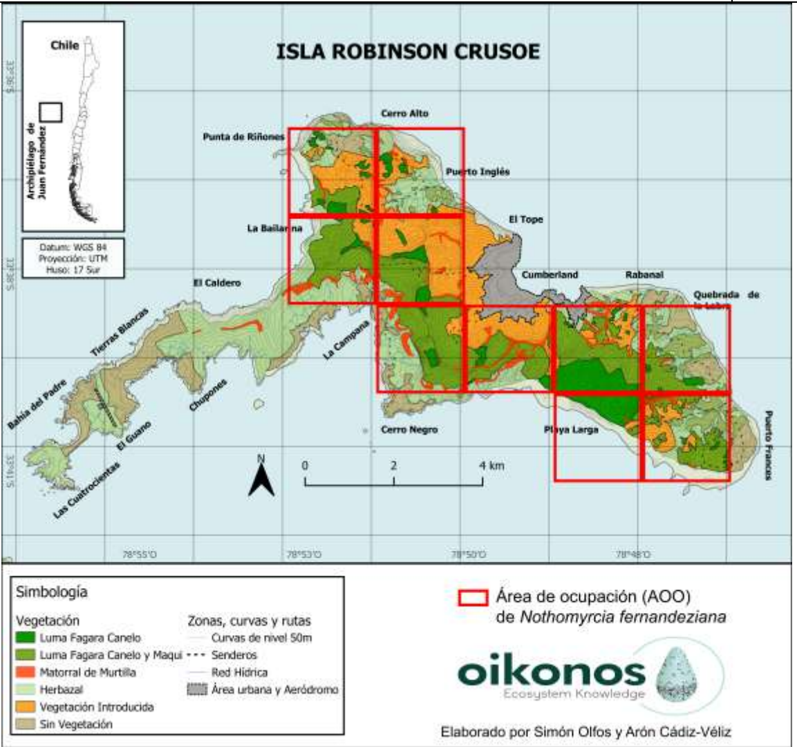
Mapa de distribución de Nothomyrcia fernandeziana . Área de ocupación (AOO): <20 Km 2 .
